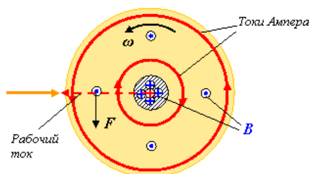
Рис. 9. Работа конструкции Родина А.Л. в режиме двигателя
