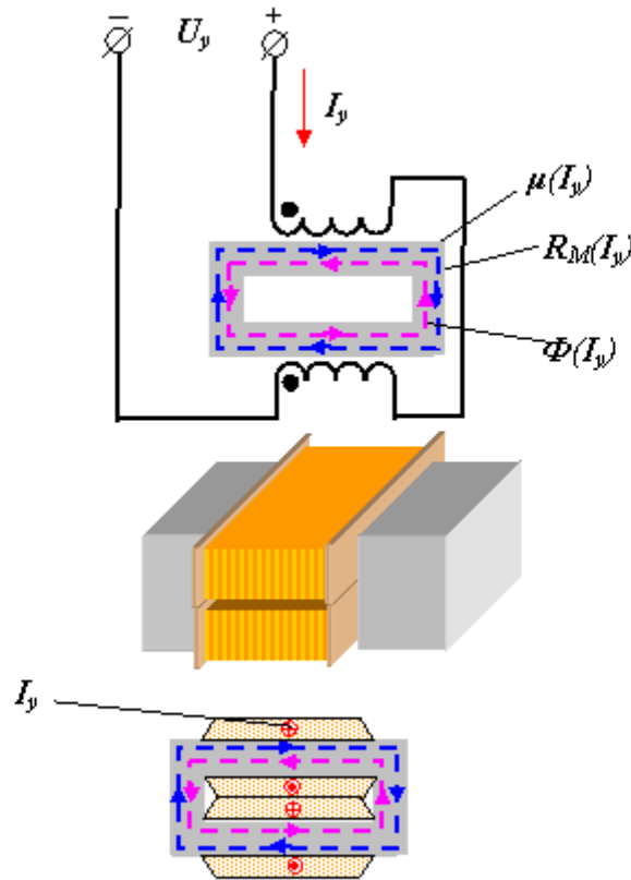
Рис. 2. Принципиальная схема, общий вид и разрез магнитного ключа МК
