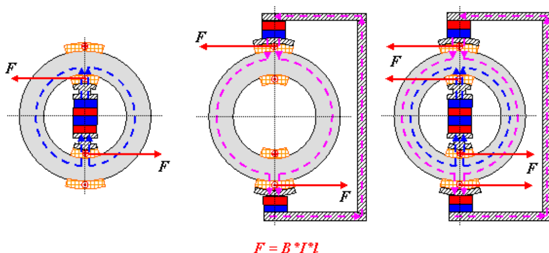
Рис. 12. Три схемы экспериментов по выявлению наличия вращательного движения с использованием обмотки типа Грамма
