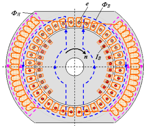
Рис. 3. Однофазный синхронный генератор с обмоткой якоря по схеме Грамма и неявнополюсным ротором (Правая и левая полу-обмотки якоря в данном положении ротора магнитных полюсов не создают)
