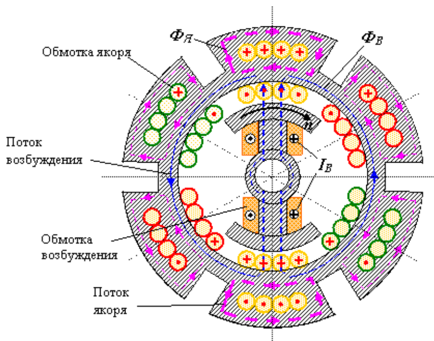
Рис. 2. Трехфазный синхронный генератор с обмоткой якоря по схеме Грамма (поперечный разрез)
