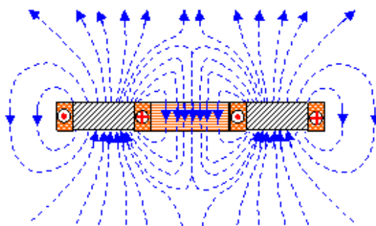
Рис. 6. Электромагнитный аналог кольцевого постоянного магнита
