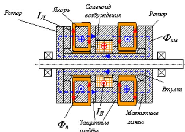
Рис. 11. Продольный разрез электродвигателя постоянного тока торцевой конструкции без коллектора и инвертора
