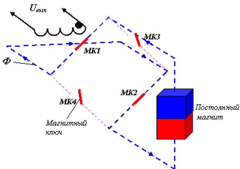
Рис. 5. Двухтактный мостовой магнито-электрический усилитель. (схема коммутации магнитных потоков)
