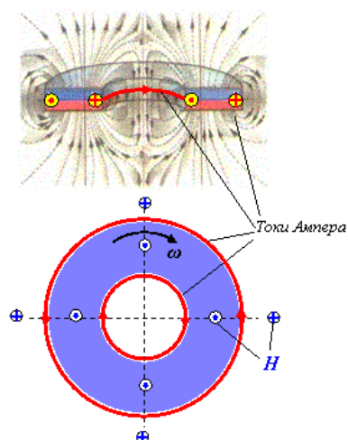
Рис. 5. Магнитное поле постоянного кольцевого магнита и его эквивалентная схема
