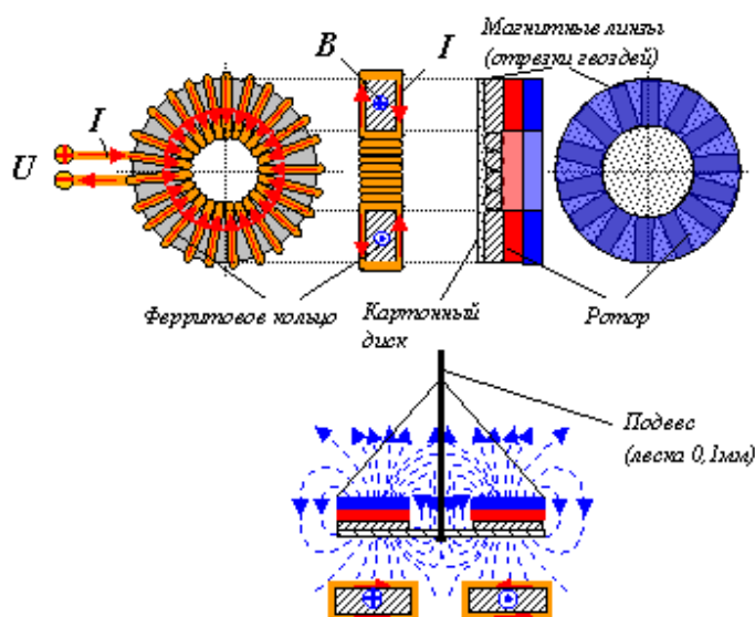
Рис. 10. Схема эксперимента по выявлению наличия вращательного движения в неподвижном магнитном поле кольцевого магнита с использованием обмотки Грамма
