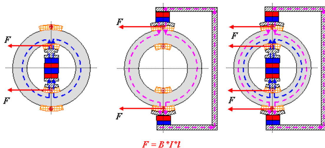
Рис. 13. Три схемы экспериментов по выявлению наличия поступательного движения с использованием обмотки типа Грамма
