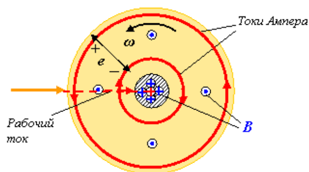
Рис. 8. Работа конструкции Родина А.Л. в режиме генератора
