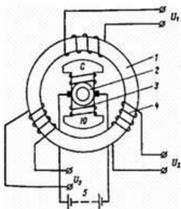
Схема синхронного генератора
